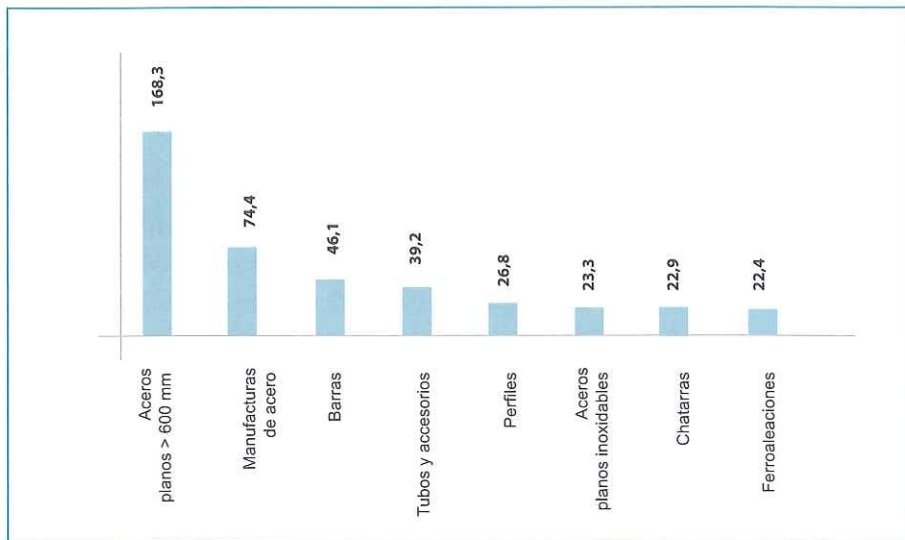
Gráfica 11. Estado de México. Productos que generan el déficit comercial en el sector del acero, 2003-2008 (millones de dólares)
